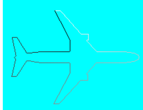
\lambda_X (679 étiquettes)
