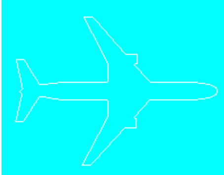
\Lambda_X (1 étiquette)
