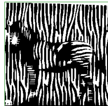
Ouverture algébrique par union des deux ensembles
