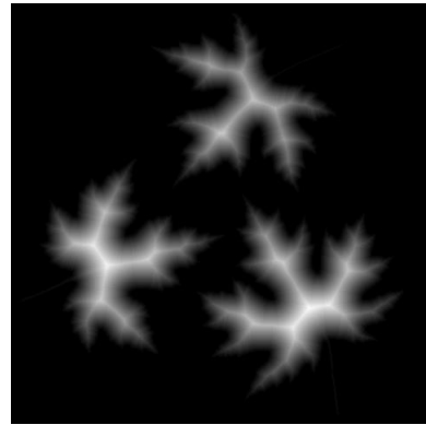
F_X^{dE}
