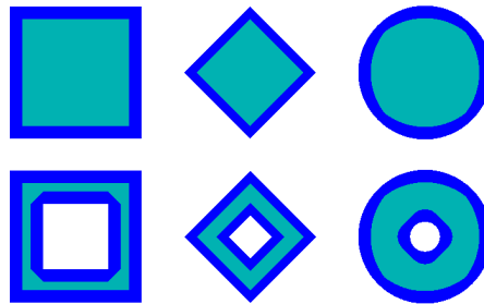
Erosion par une boule de d_4
