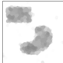
\Xi_5
