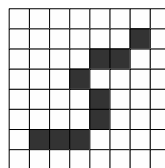
Un chemin 8-connexe
