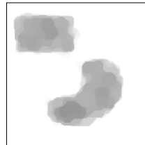
\Xi_8
