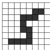
Un chemin 4-connexe
