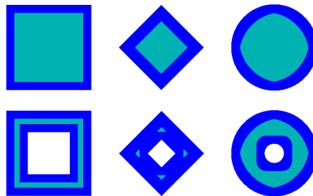
Erosion par une boule de d_8
