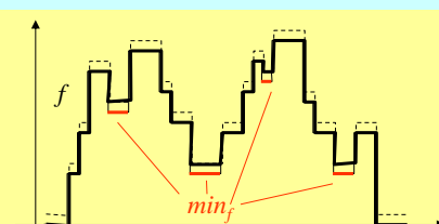
Minima régionaux : par dualité
