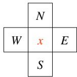
dénomination cardinale des 4-voisins
