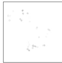
Application directe du filtre alterné \gamma_4 \phi_4
