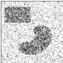
\Xi_1
