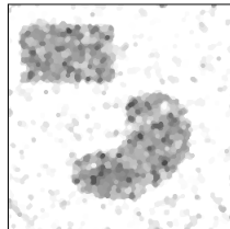
\Xi_2
