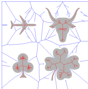
Sk_5(X)
