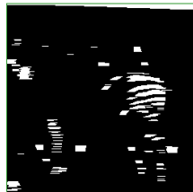
Ouverture morphologique par un segment horizontal
