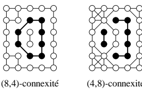
(8,4)-connexité
