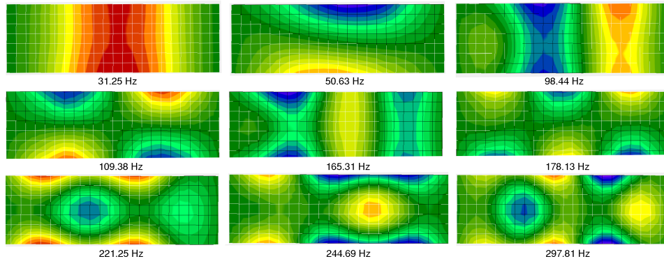
FIGURE 4 – Déformées modales de la plaque d'aluminium encadrée sur deux bords
